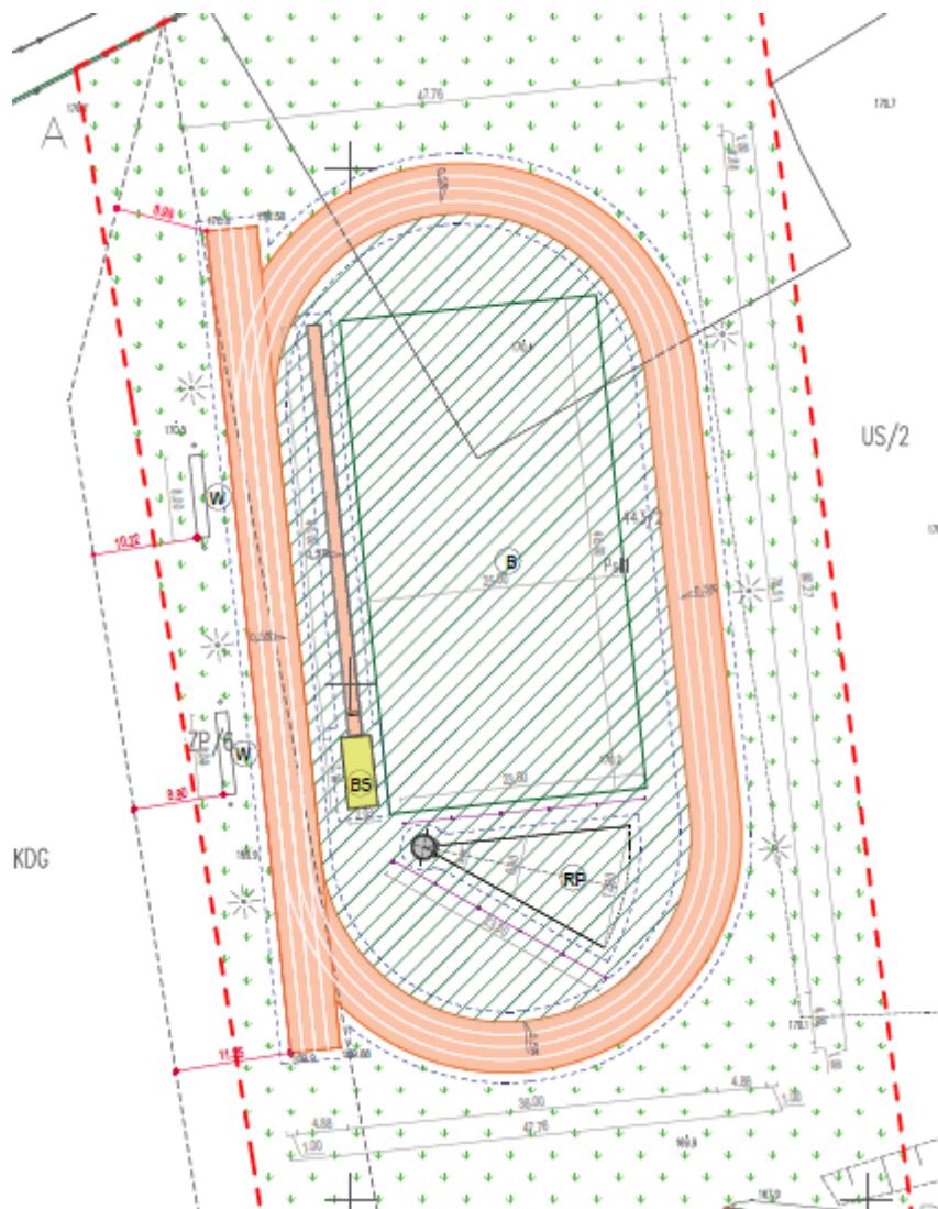
Wizualizacja boiska lekkoatletycznego przy Stadionie Miejskim
